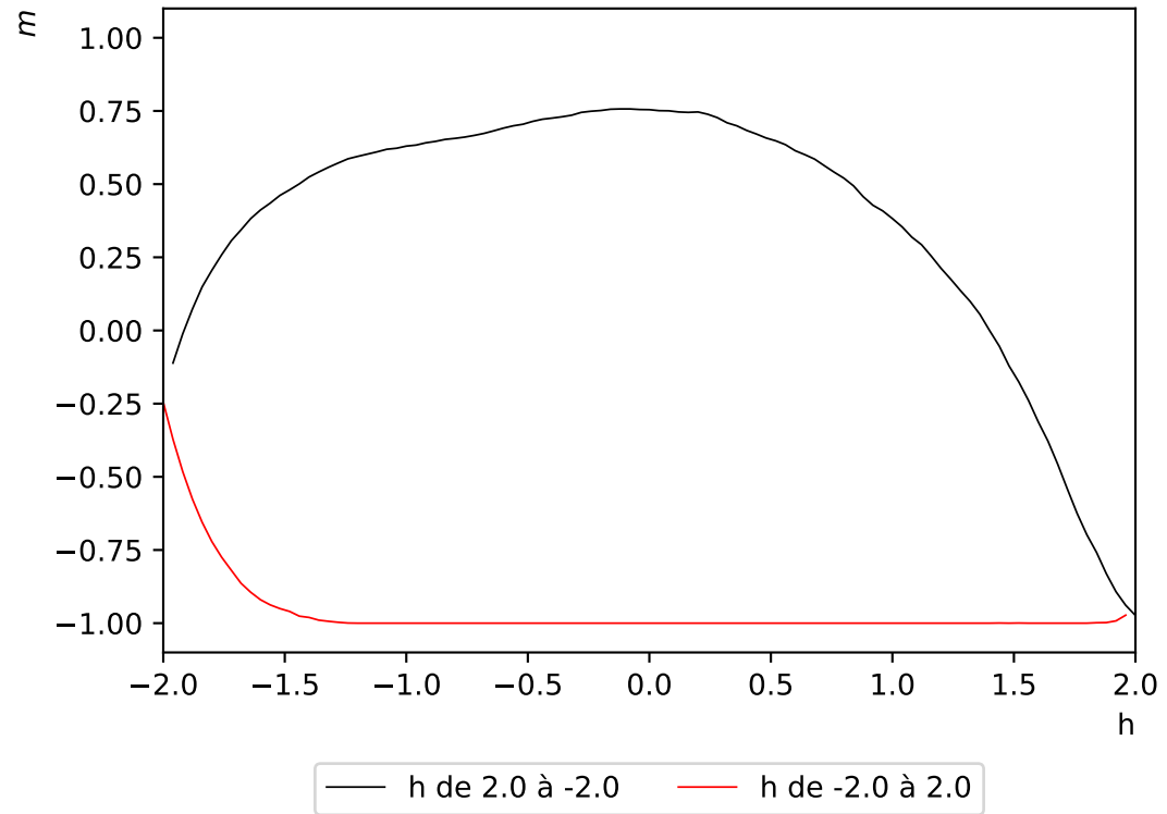
Hystérésis de l'aimantation - réseau de taille L=64 - champ magnétique d'amplitude h=2 à T=0.5
